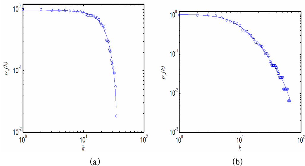
图 15 网络的累积度分布. (a) 科学部网络; (b) 申请单位网络。
