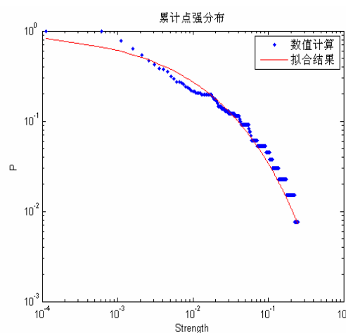
图 6 基金面上网络累积点强分布图。
