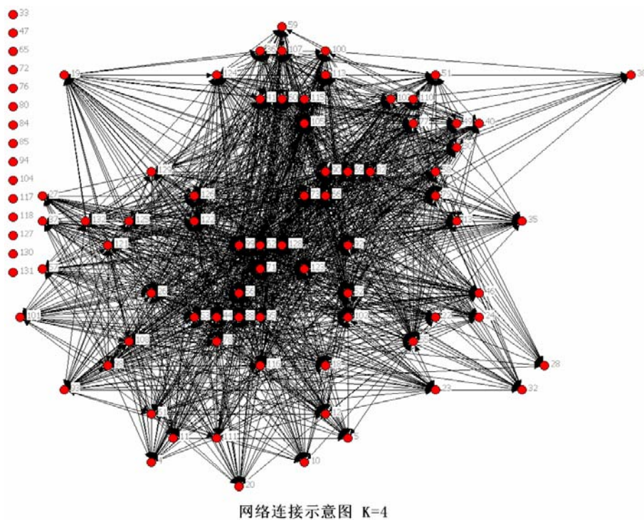
(c) K=4 情形。
