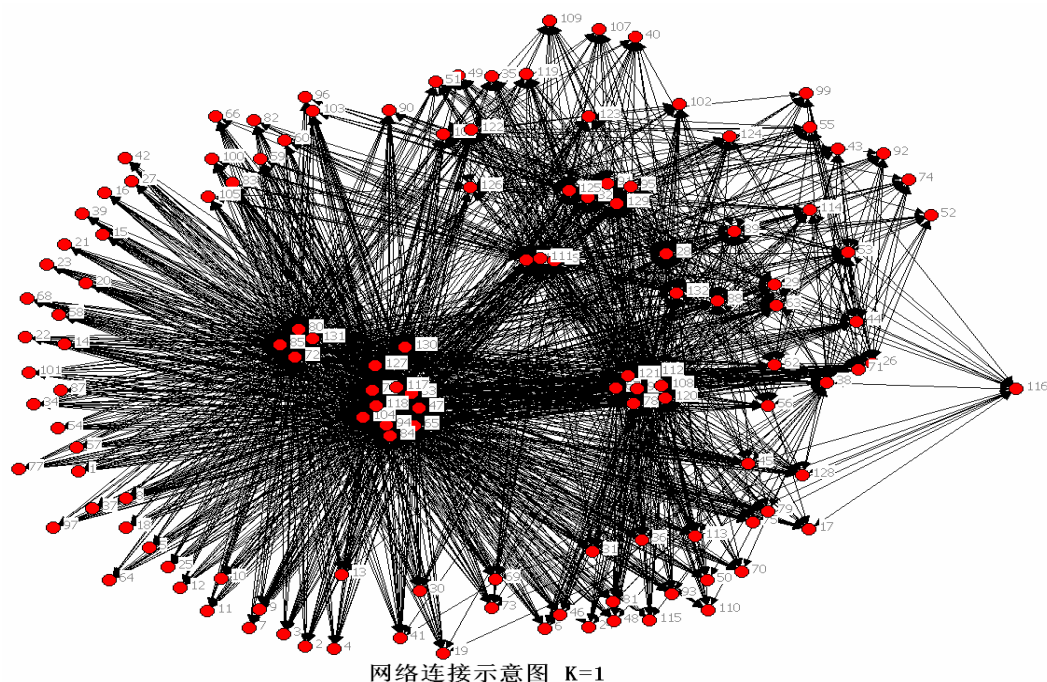
(a) K=1 情形。
