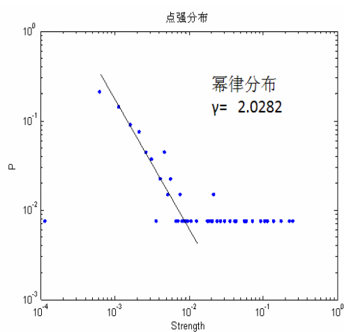
图 5 基金面上网络点强分布图。
