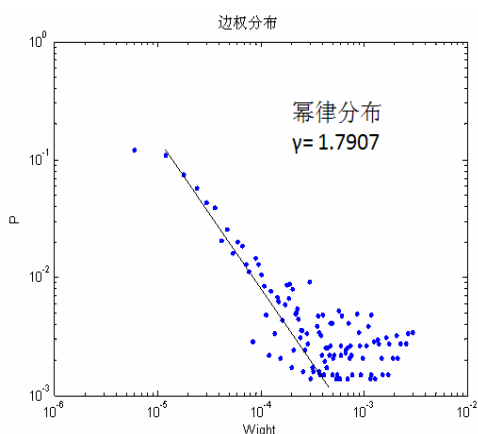
图 7 基金面上网络边权分布。
