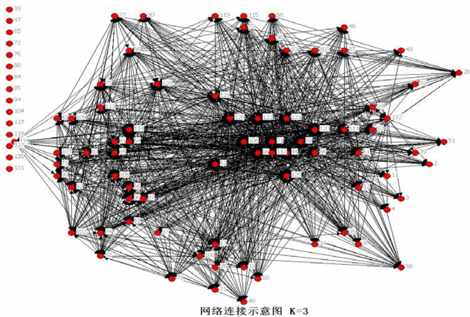
(b) K=3 情形。
