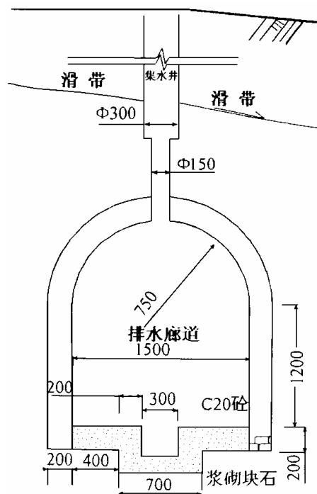
图3 滑坡地下排水廊道剖面示意图
