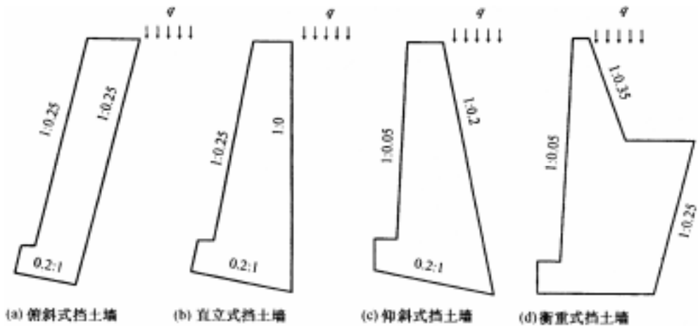
图10 重力挡墙断面一般型式图
