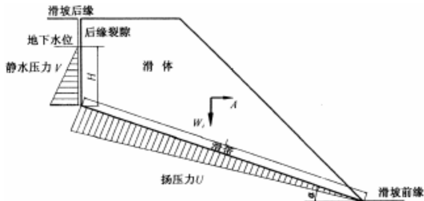
图 A.3 极限平衡法 (岩质滑坡计算模型)
