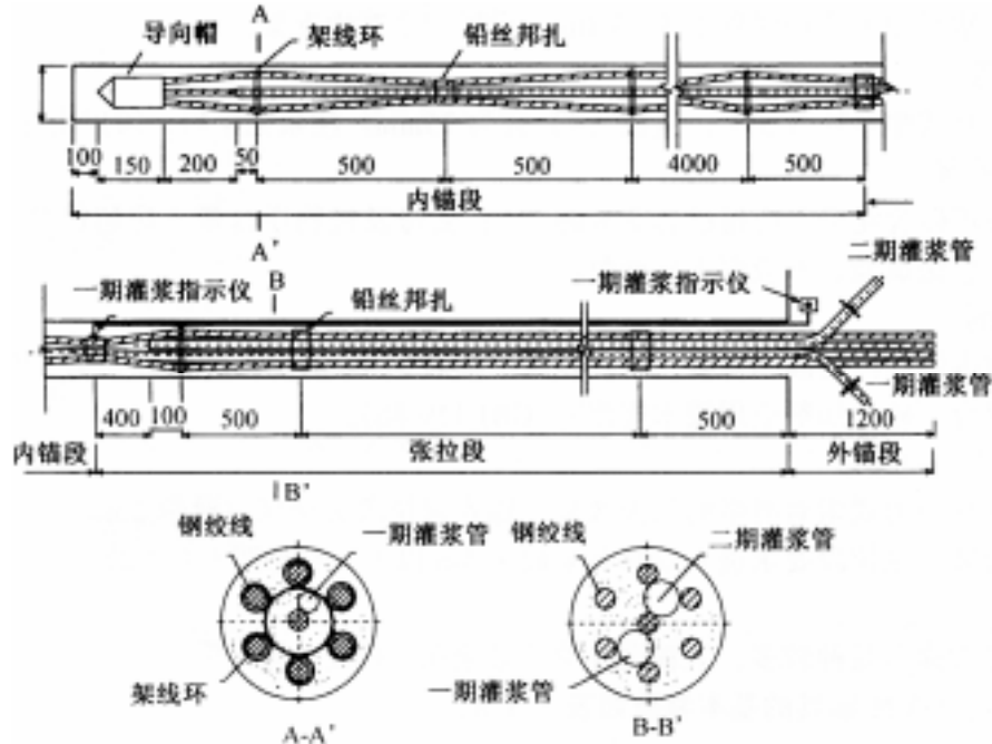
图5 1000kN 级预应力锚索结构图
