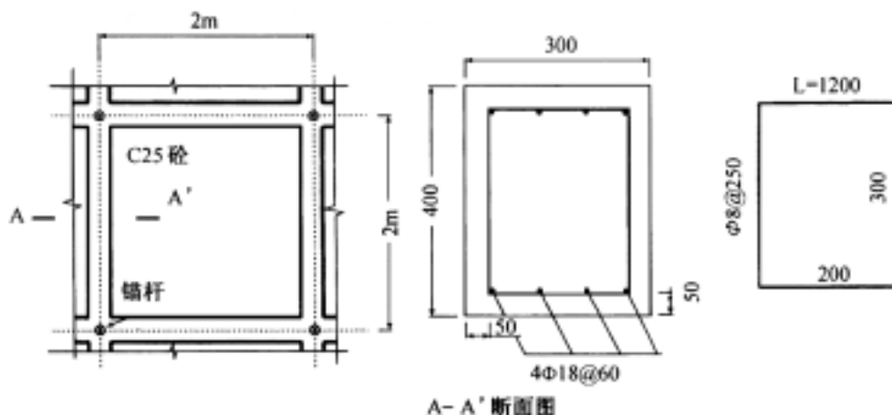
图9 现浇钢筋砼格构断面图
