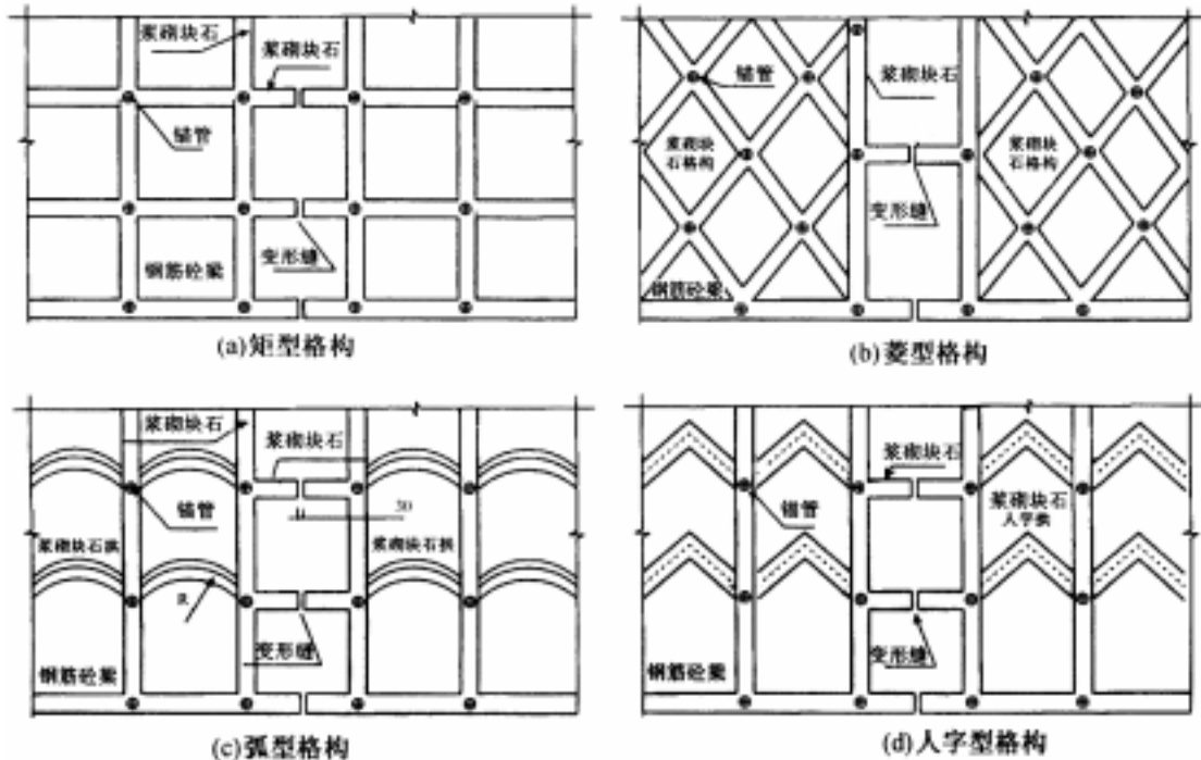
图7 格构平面布置型式图
