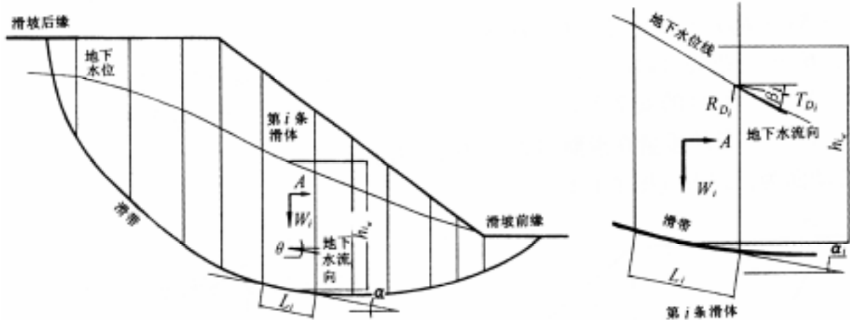
图 A.1 瑞典条分法(圆弧形滑动面)(堆积层滑坡计算模型之一)
