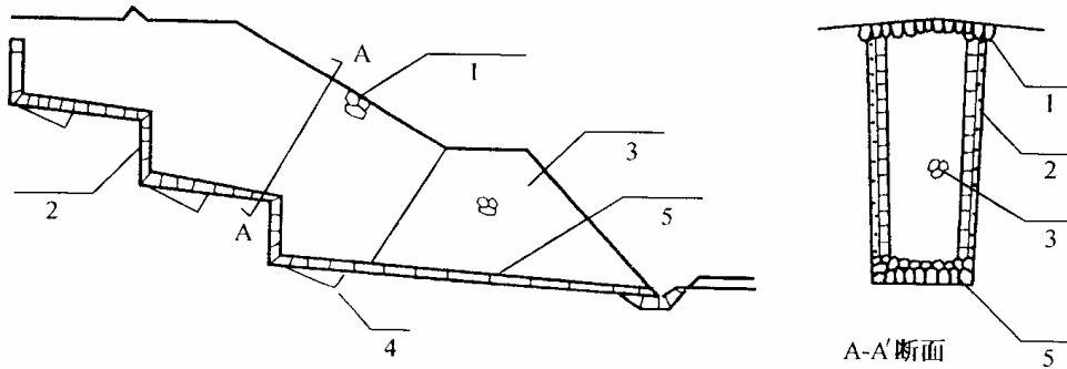
注：1、大块干砌片石；2、反滤层；3、干砌片石；4、浆砌片石；5、牙石 图2 滑坡地下排水支撑盲沟断面示意图
