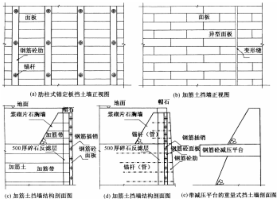
图11 锚定板、加筋土和减压平台挡土墙型式图
