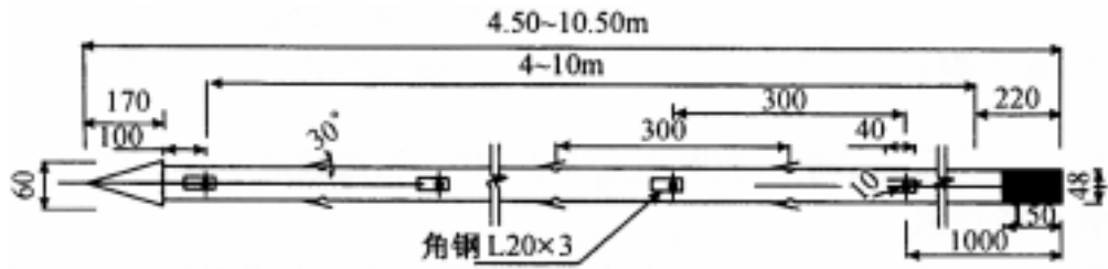
图8 格构锚管结构图
