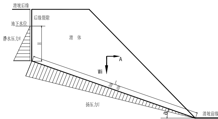
图 E.3 岩质滑坡计算模型：极限平衡法
