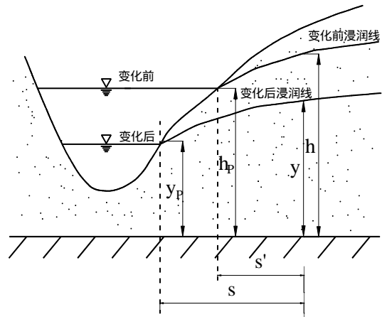
图 F.1 地表水位变化引起的岸坡地下水稳定运动
