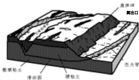
E.滑动(Slide)
