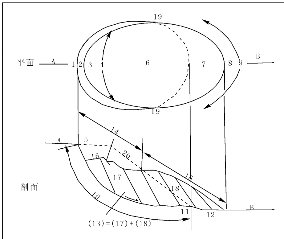
图 A.1 滑坡要素图
